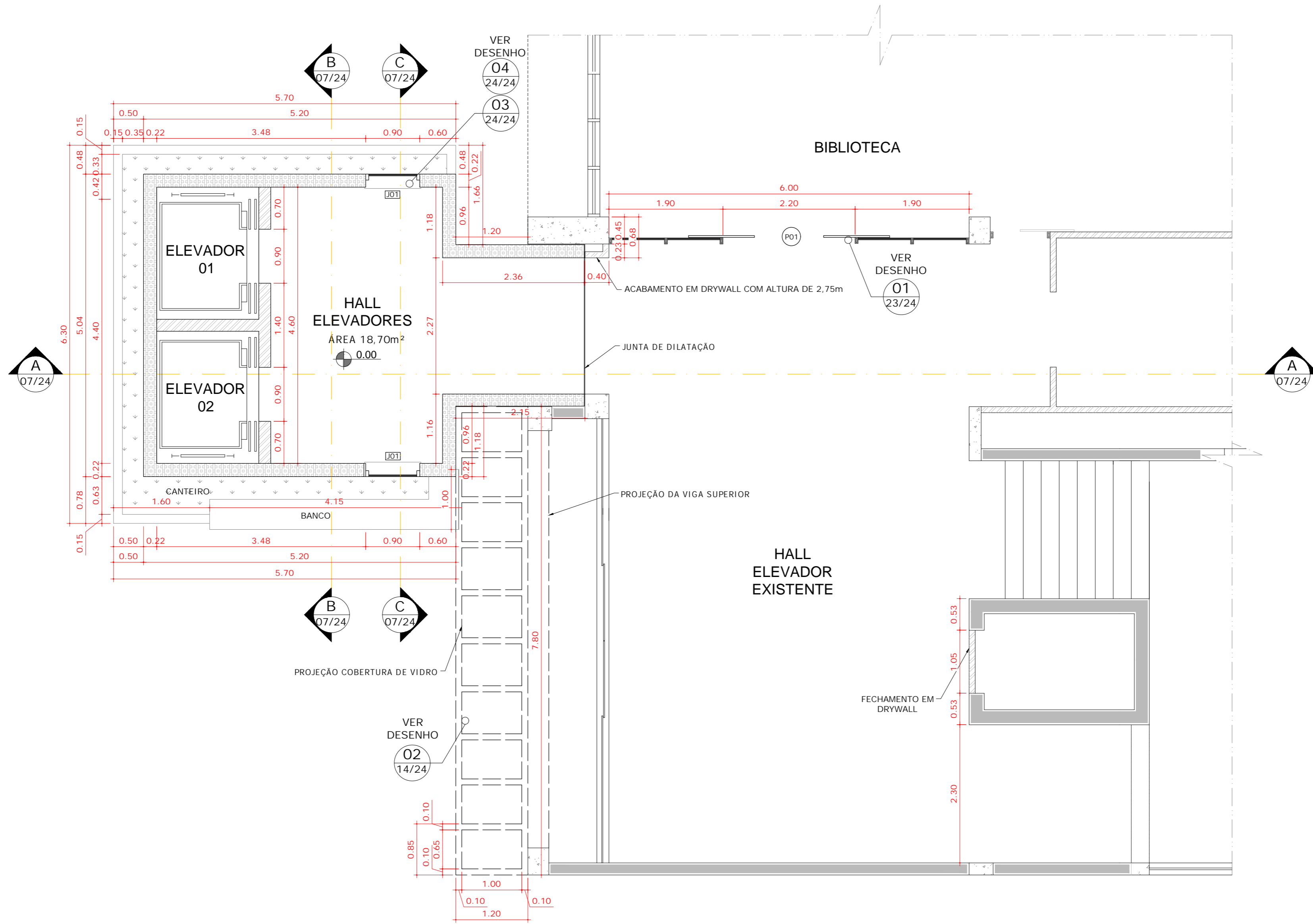
01 PLANTA ELEVADOR- PAV. 1 ESCALA 1:50
