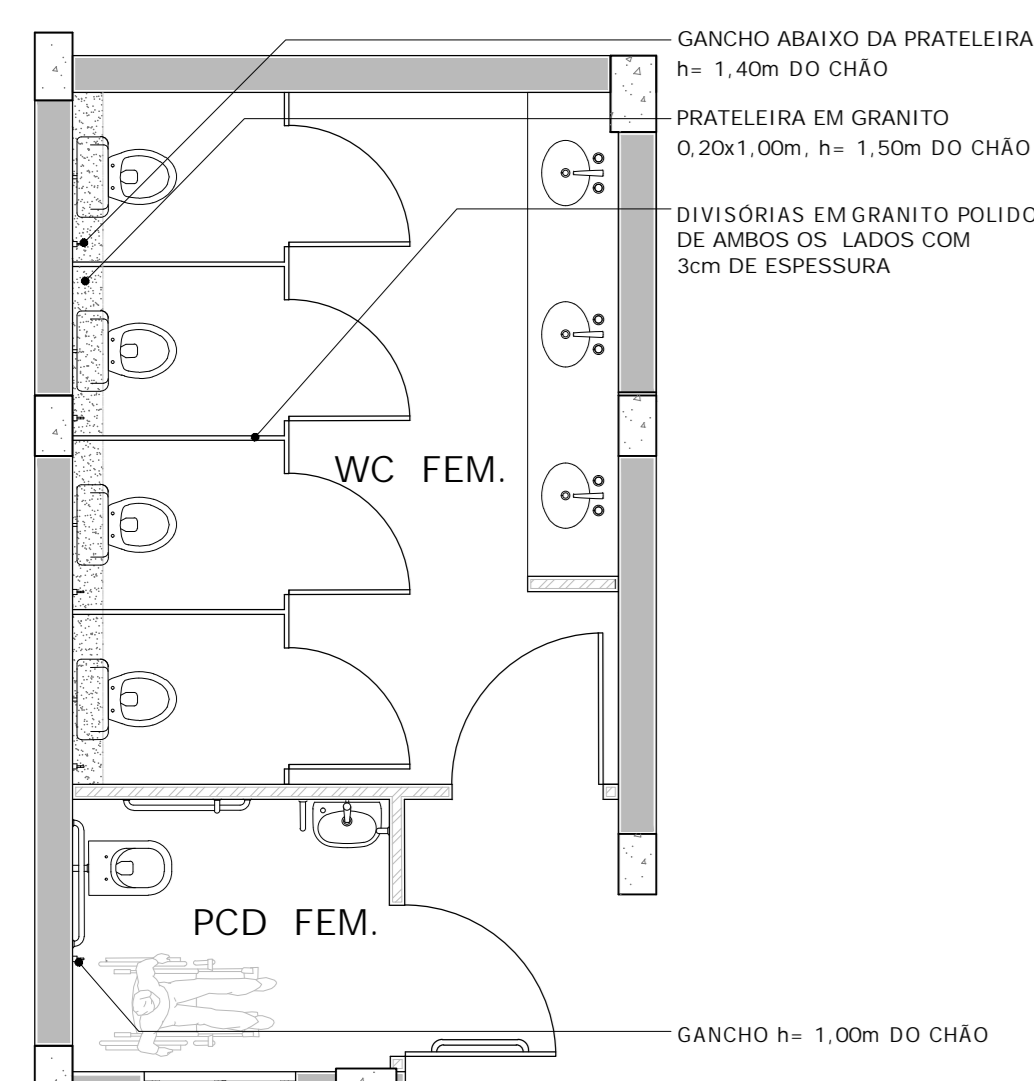
01 PLANTA- BANHEIROS FEM. ESCALA 1:50
