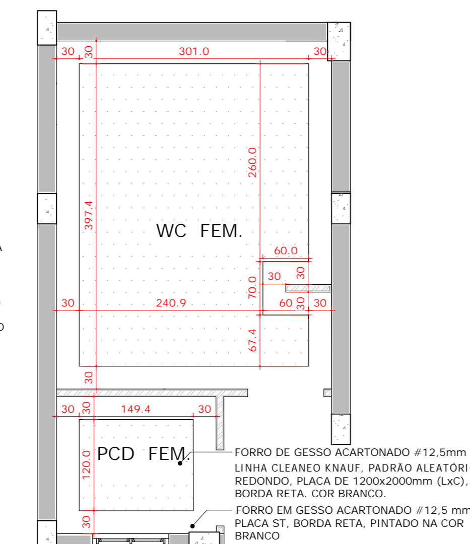
03 PLANTA DE FORRO - WC. FEM. ESCALA 1:50
