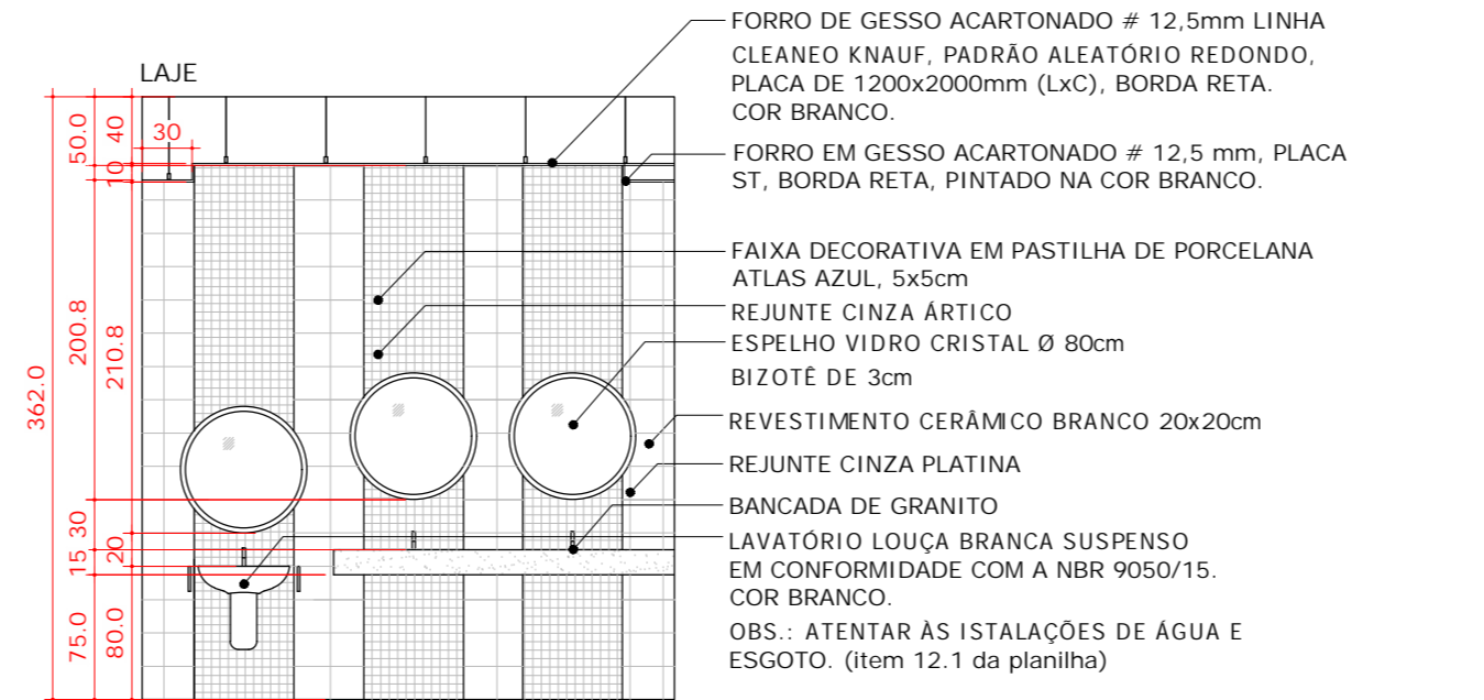
05 VISTA- ESPELHOS BANHEIRO FEM. ESCALA 1:50
