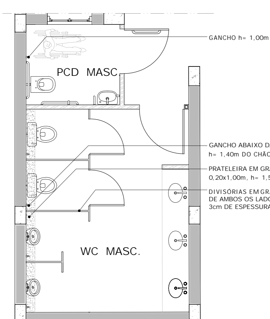
02 PLANTA- BANHEIROS MASC. ESCALA 1:50
