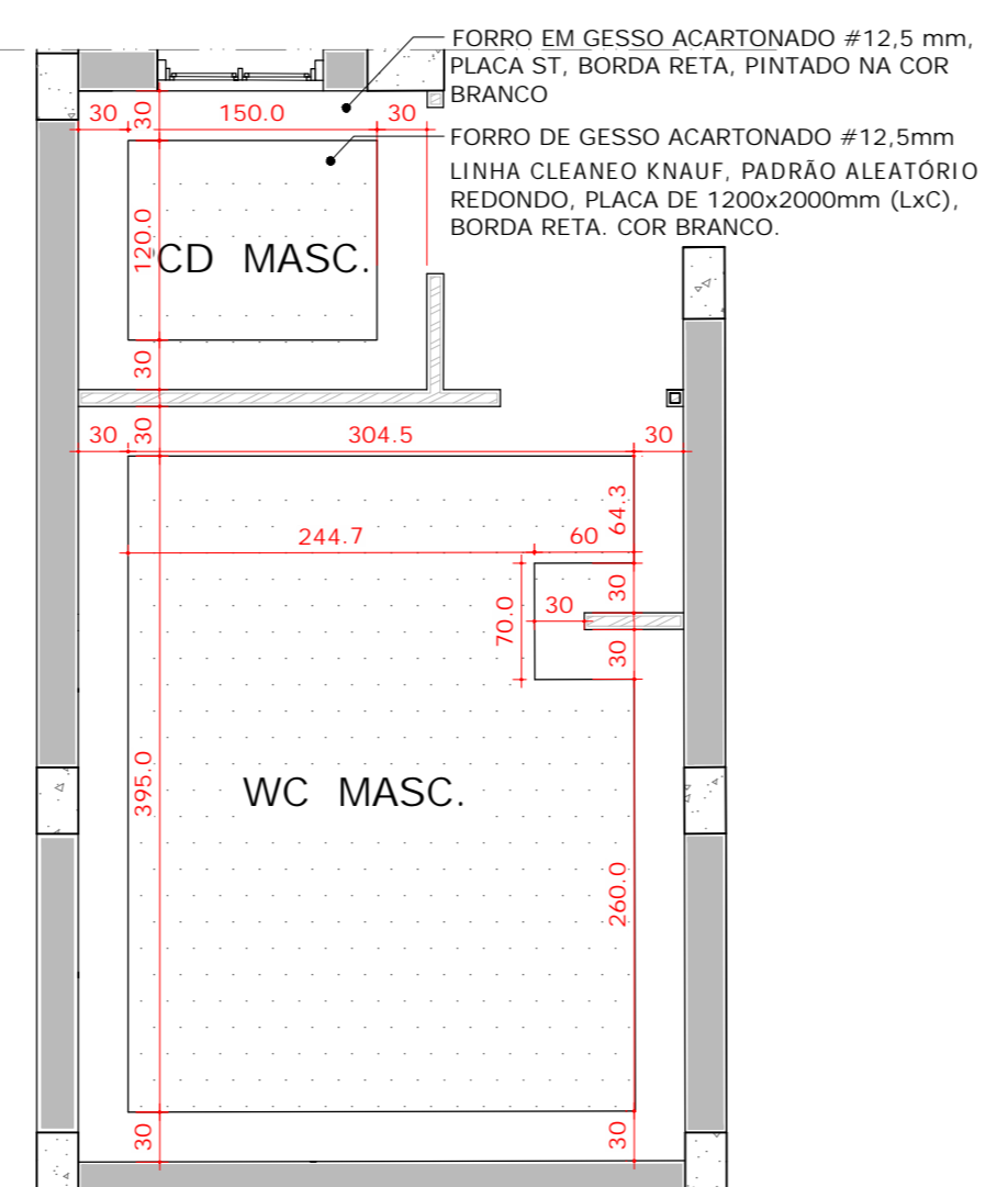
04 PLANTA DE FORRO - WC. MASC ESCALA 1:50
