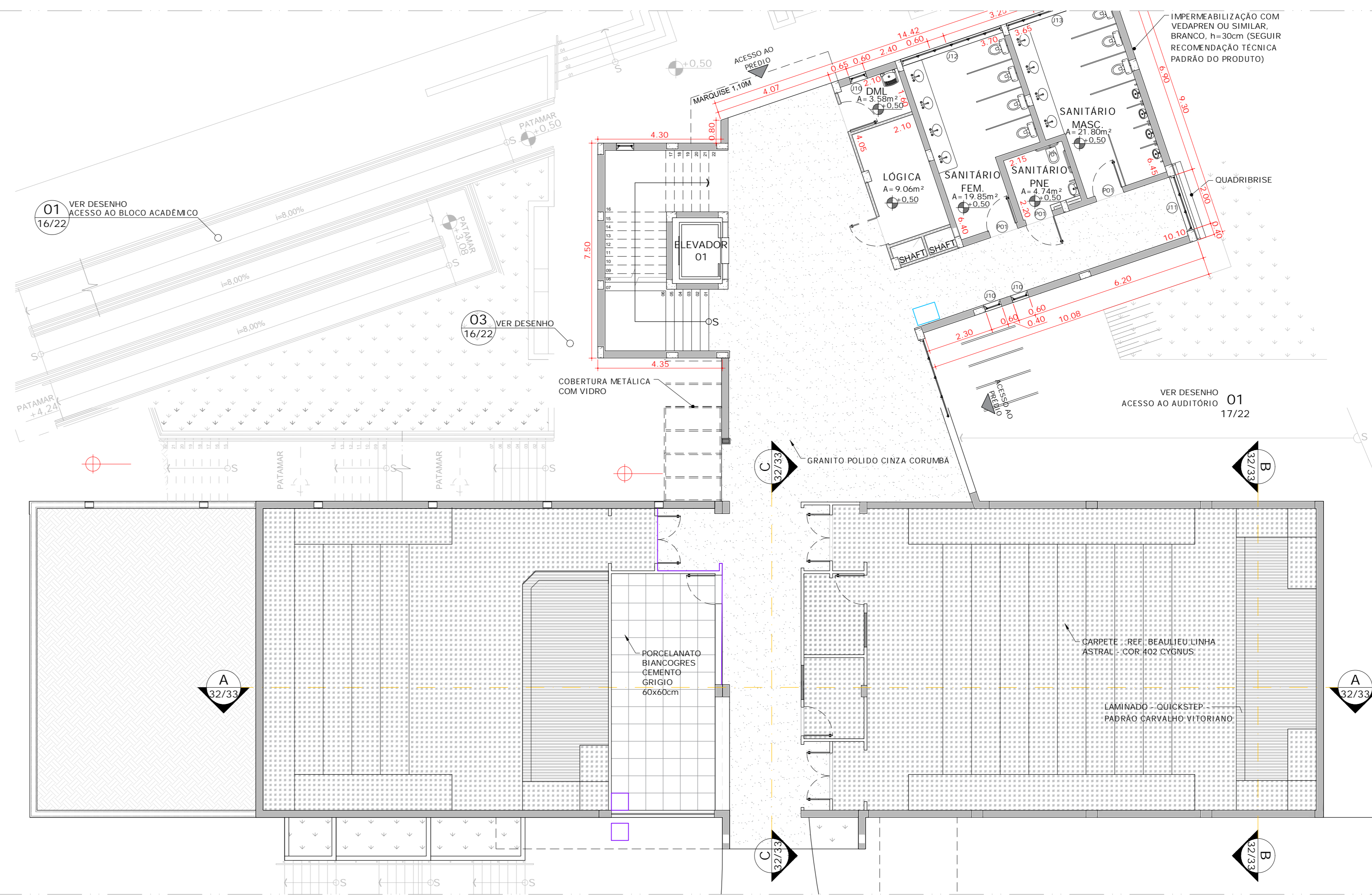
03 PLANTA REVESTIMENTOS PISO ESCALA 1:100
