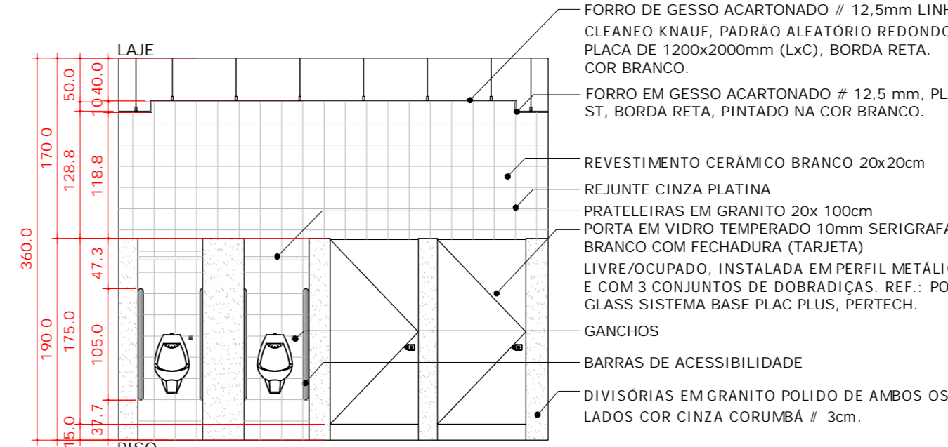
08 VISTA- CABINES BANHEIRO MASC. ESCALA 1:50
