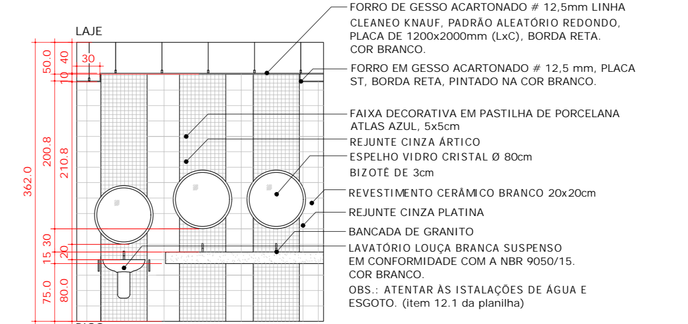
06 VISTA- ESPELHOS BANHEIRO MASC. ESCALA 1:50
