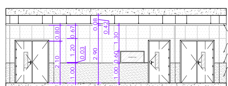
06 CORTE CC' ESCALA 1:100
