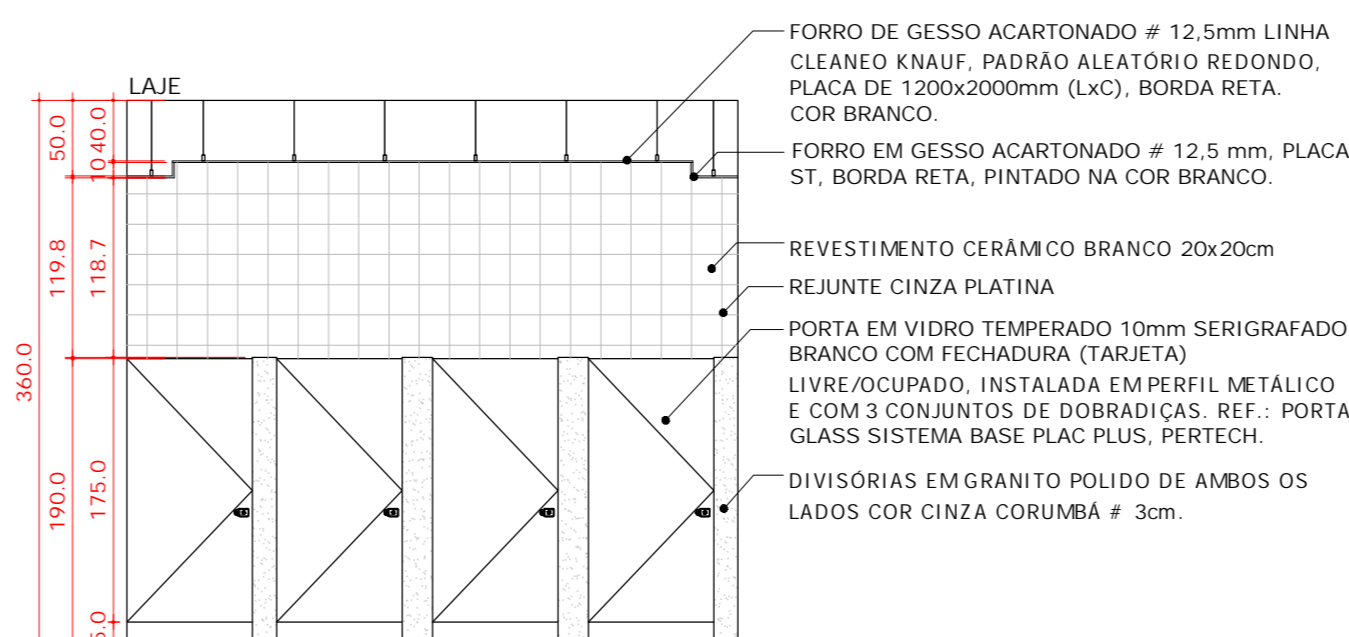
07 VISTA- CABINES BANHEIRO FEM. ESCALA 1:50
