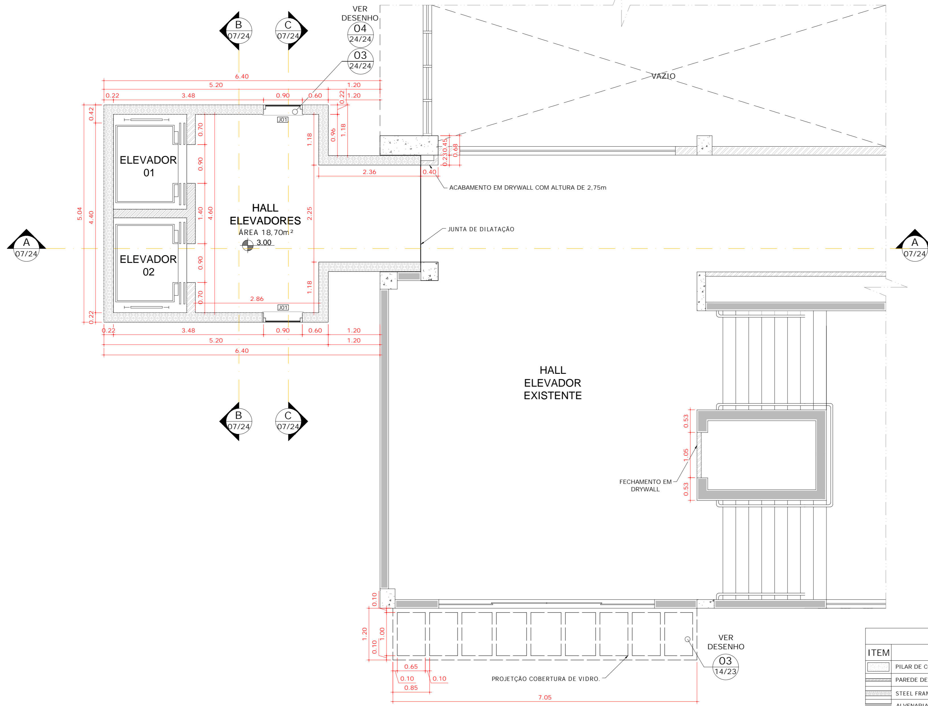
01 PLANTA ELEVADOR - PAV. 2 ESCALA 1:50
