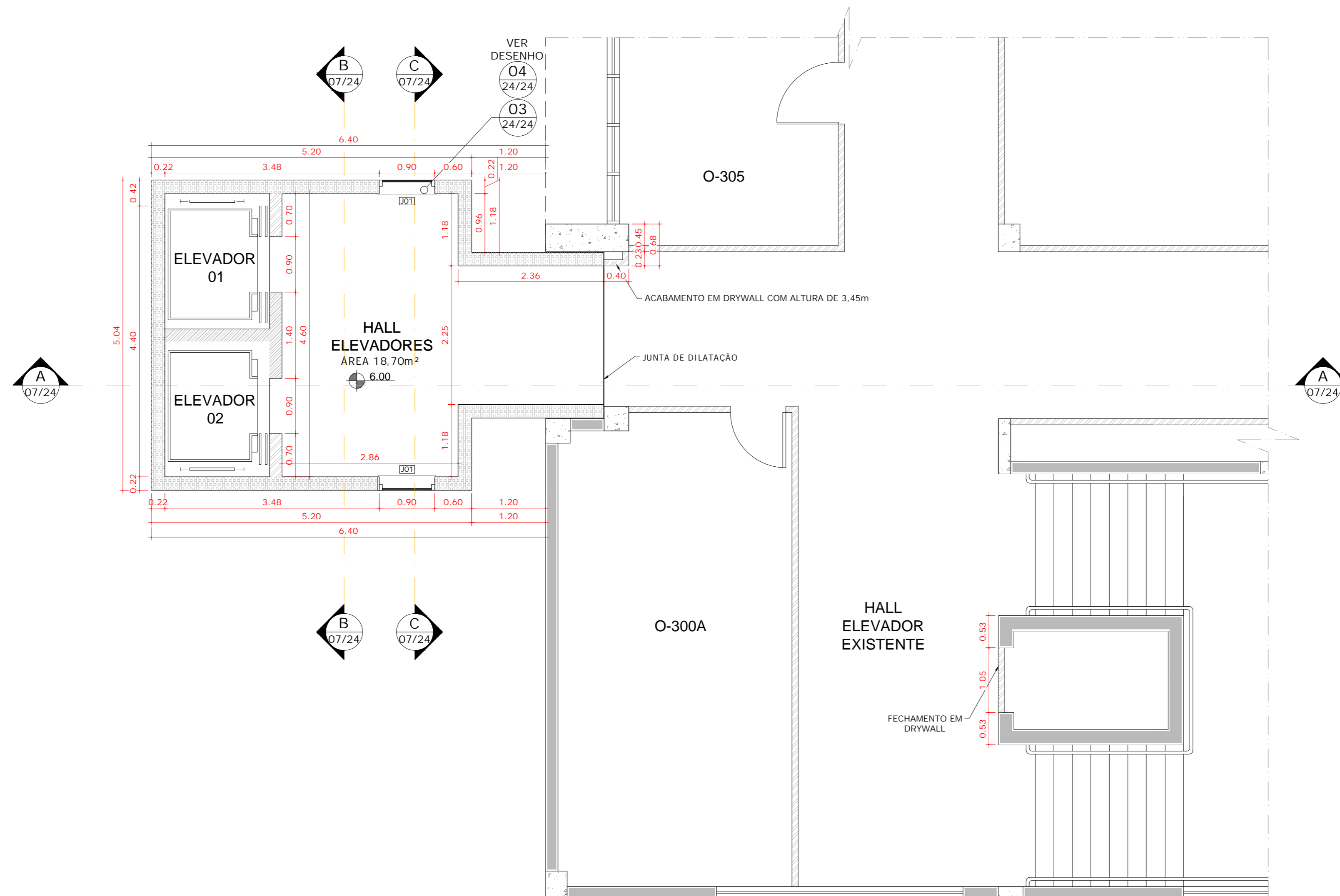
01 PLANTA ELEVADOR - PAV. 3 ESCALA 1:50
