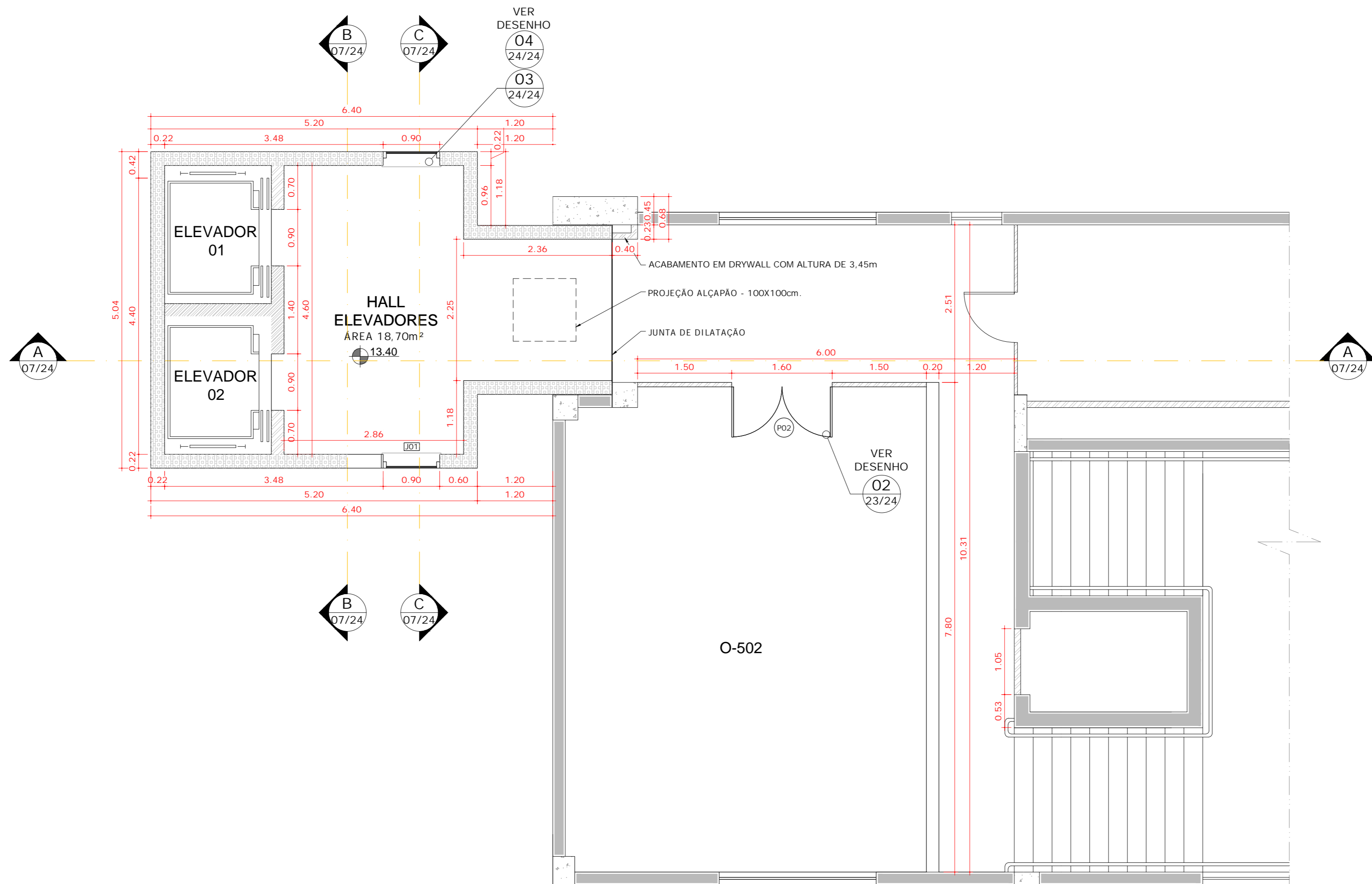
01 PLANTA ELEVADOR - PAV. 5 ESCALA 1:50
