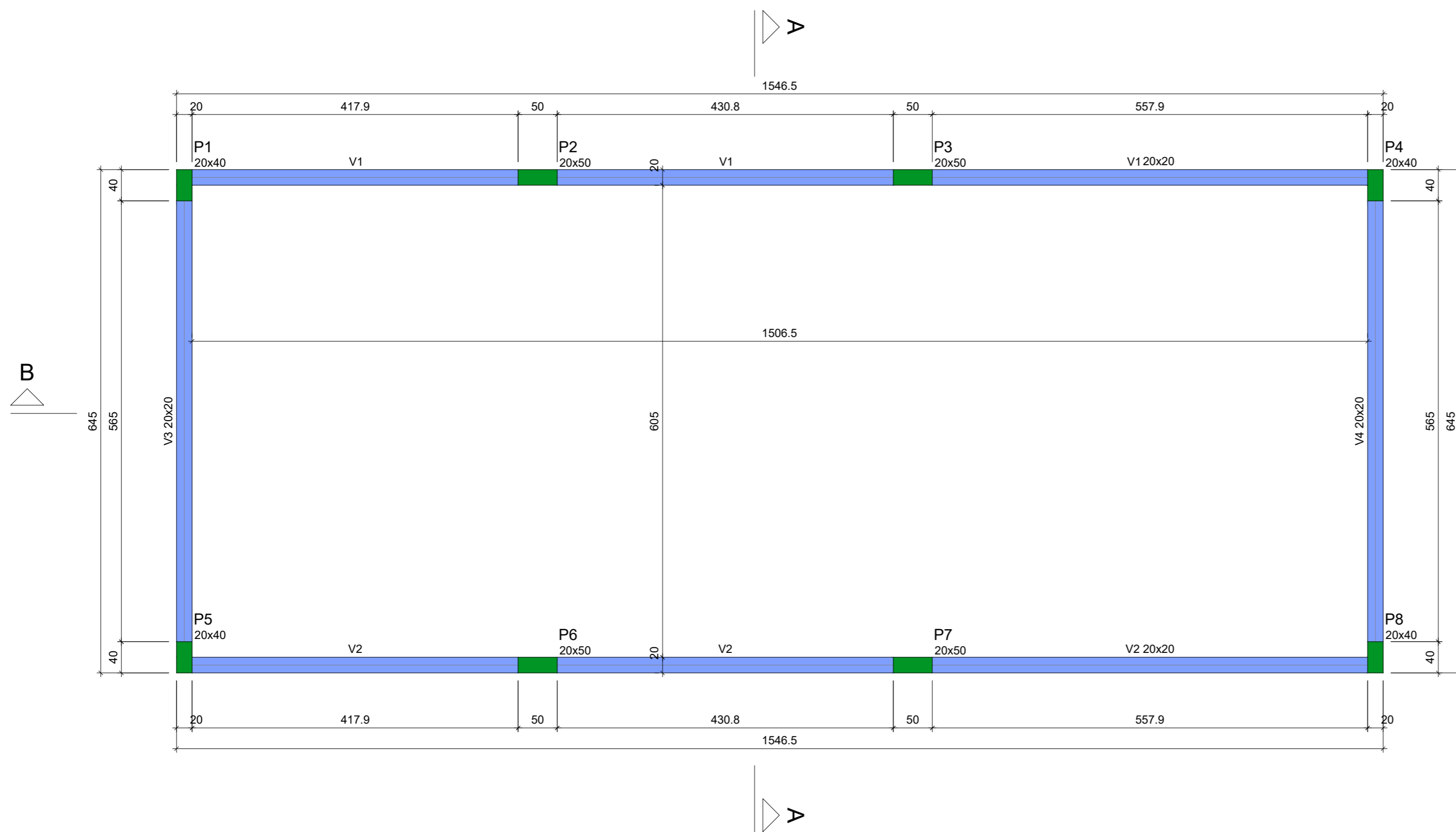
PLANTA DE FORMAS DO RESPALDO - NÍVEL 500 Escala 1:50
