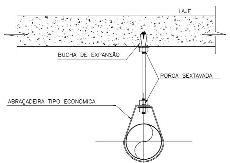
02 SUPORTE NA LAJE. ESCALA: S/ ESC.
