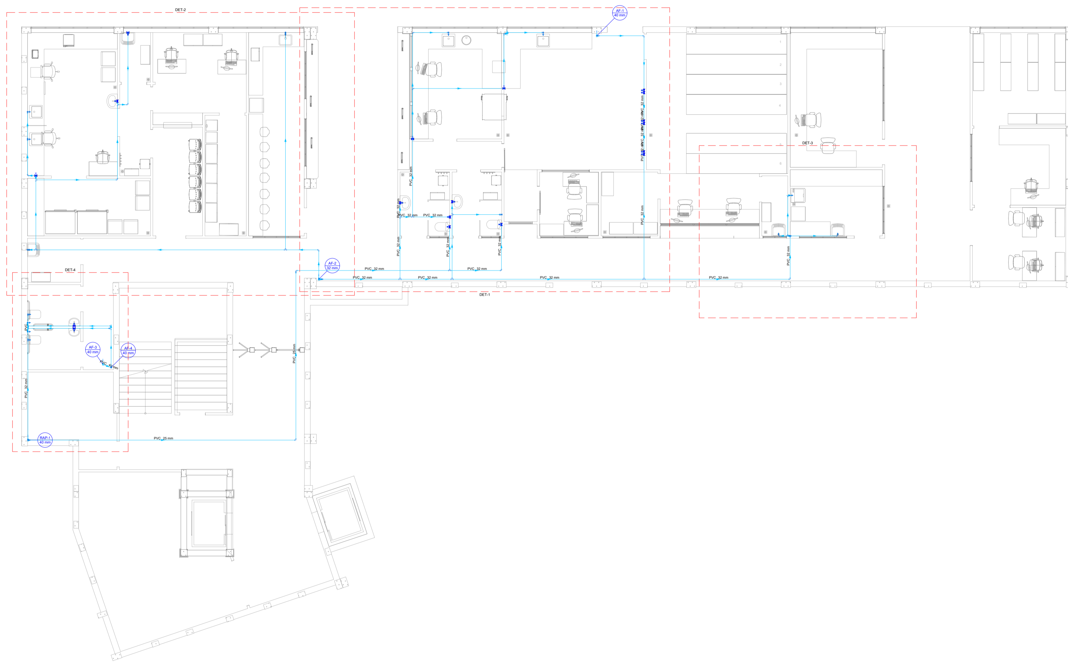
Projeto hidráulico do Piso 1 - Nível +0,50 Escala 1:100
