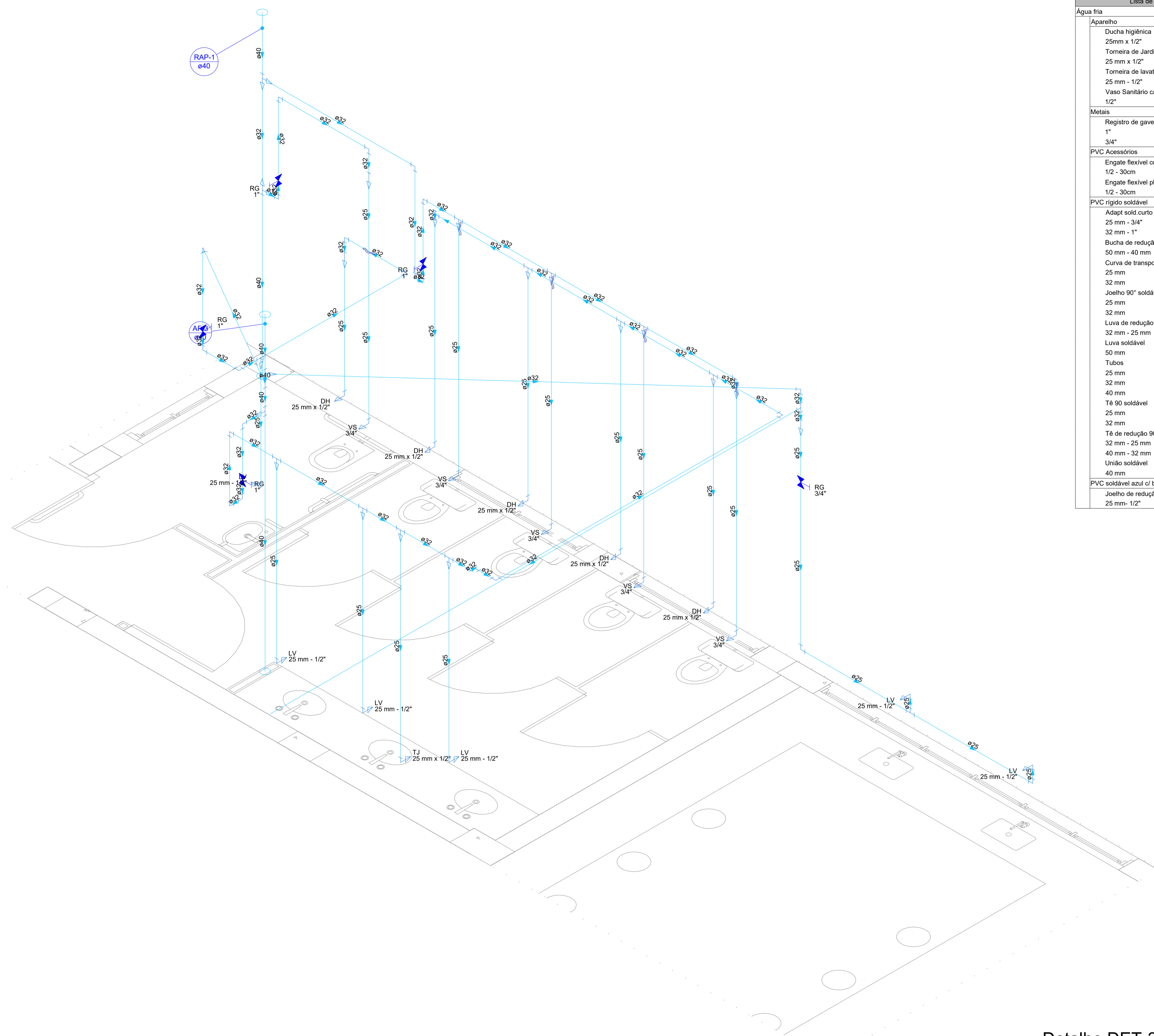
Detalhe DET-31 Escala 1:25
