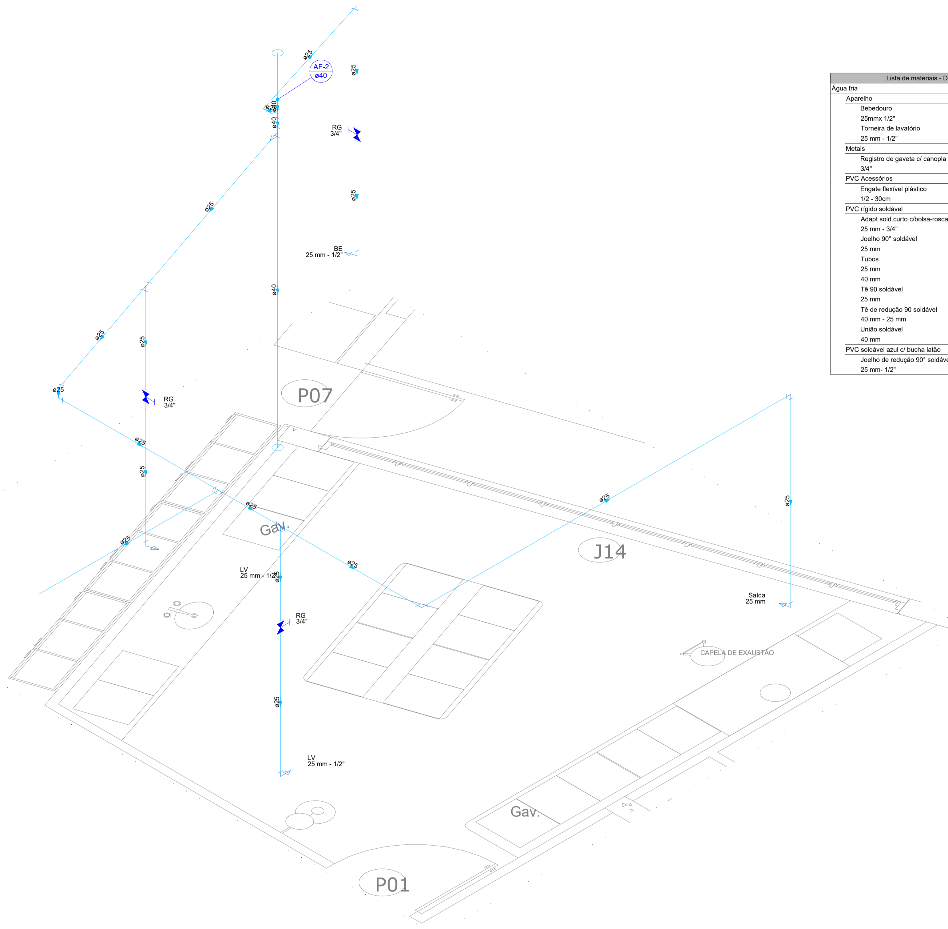
Detalhe DET-3 Escala 1:25
