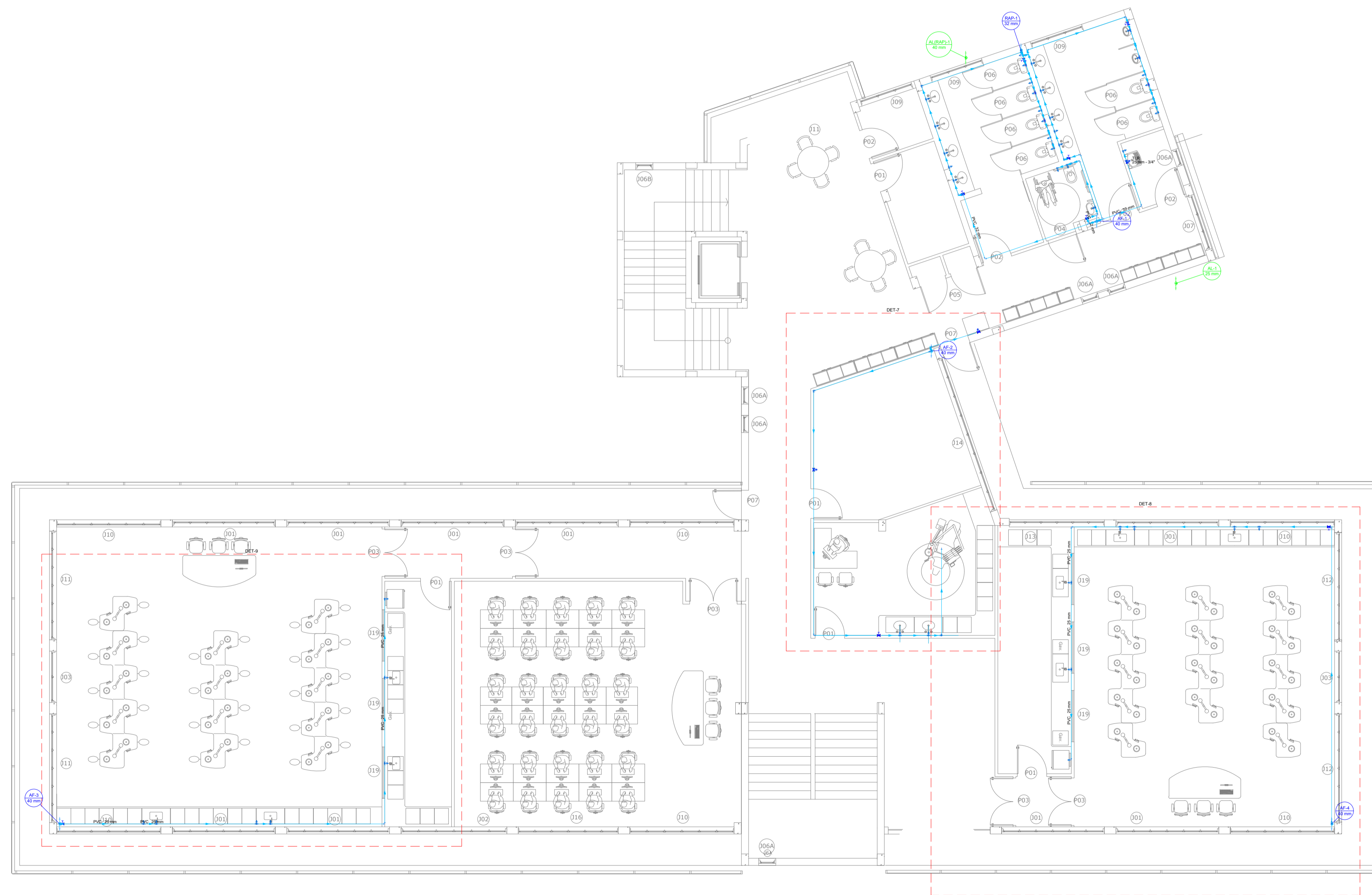
Projeto hidráulico do Piso 3 - Nível +7,98 Escala 1:100
