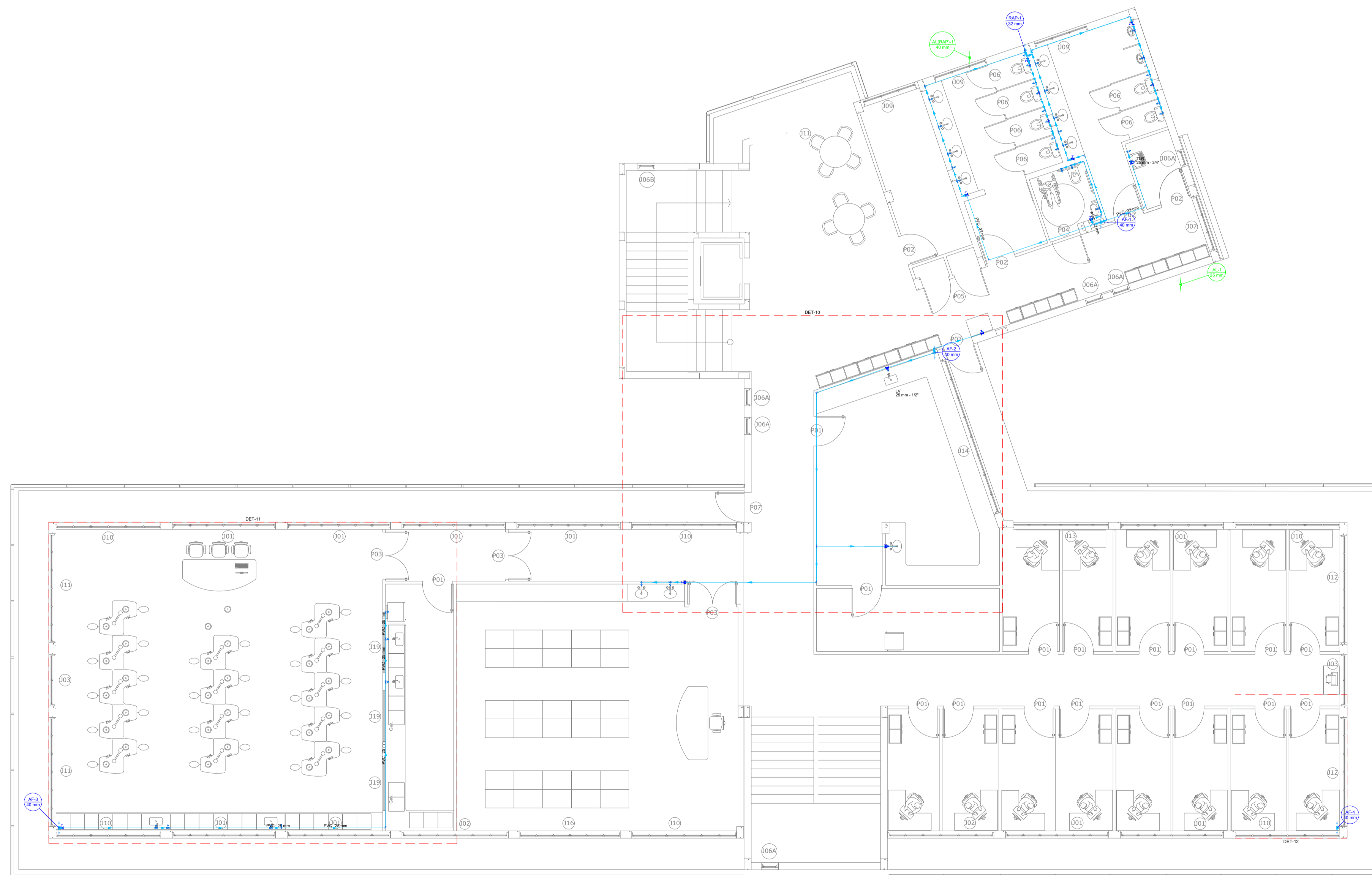
Projeto hidráulico do Piso 4 - Nível +11,72 Escala 1:100
