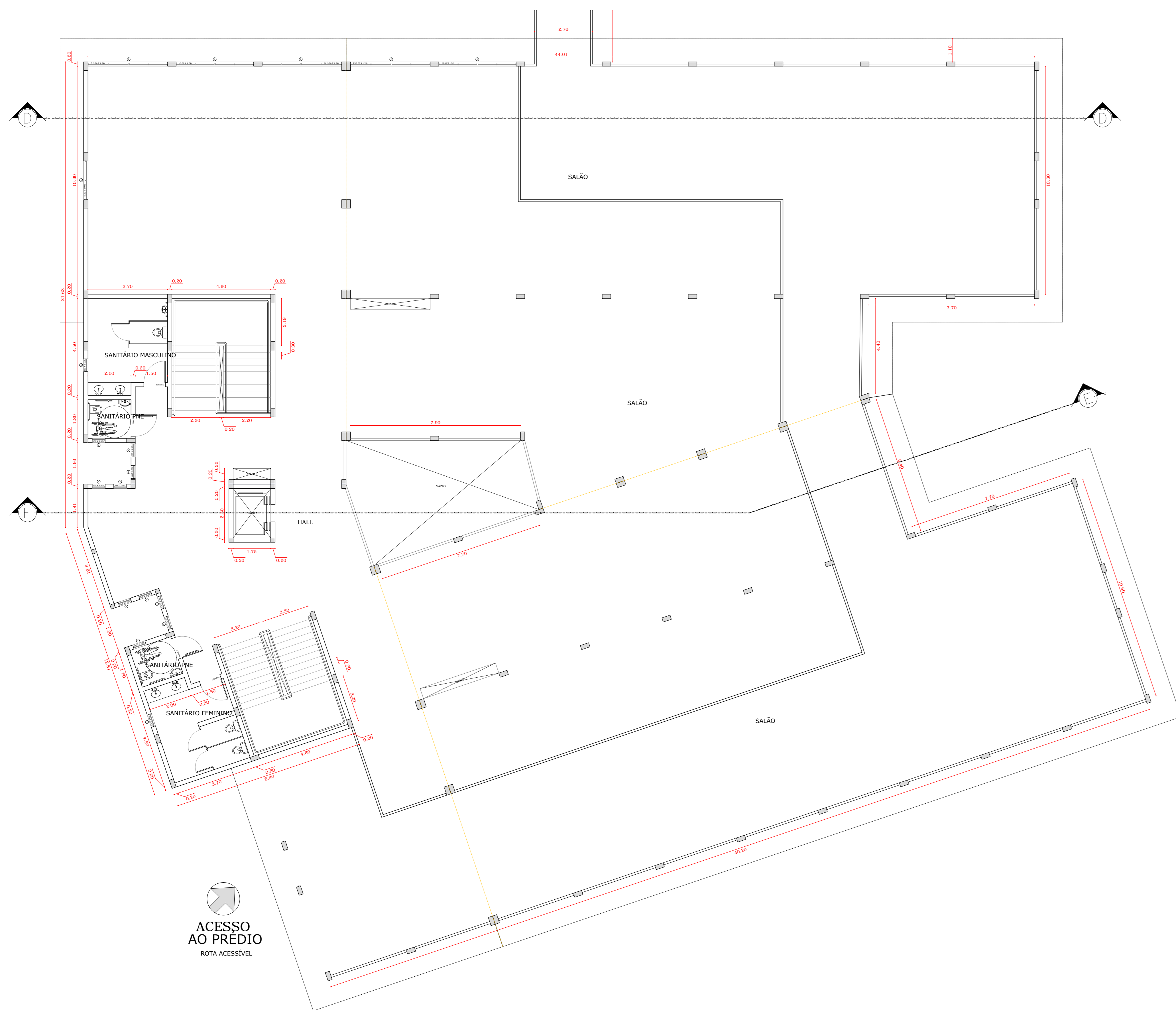
12 PISO 3 ESCALA 1:100
