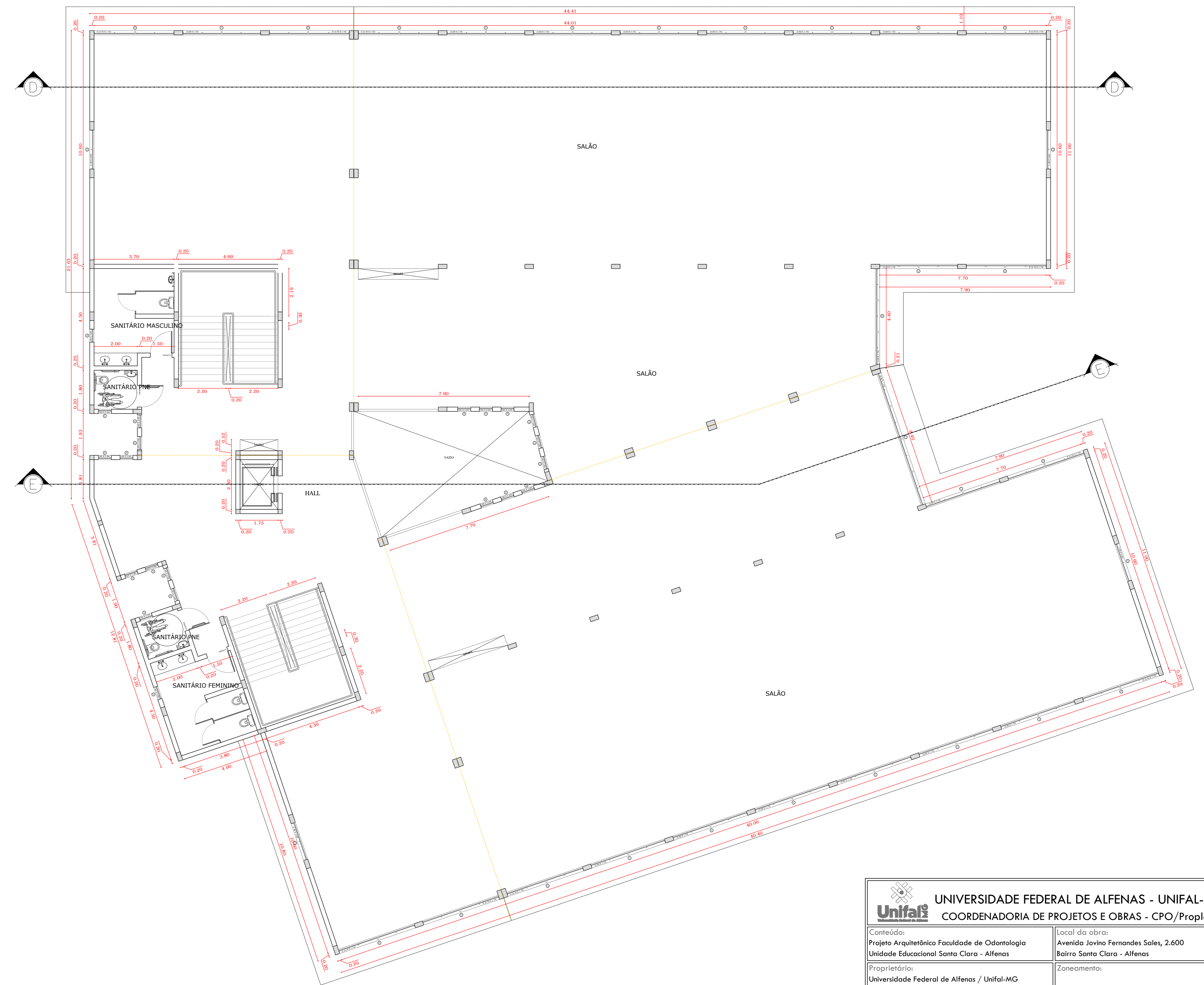
15 PISO 6 ESCALA 1:100
