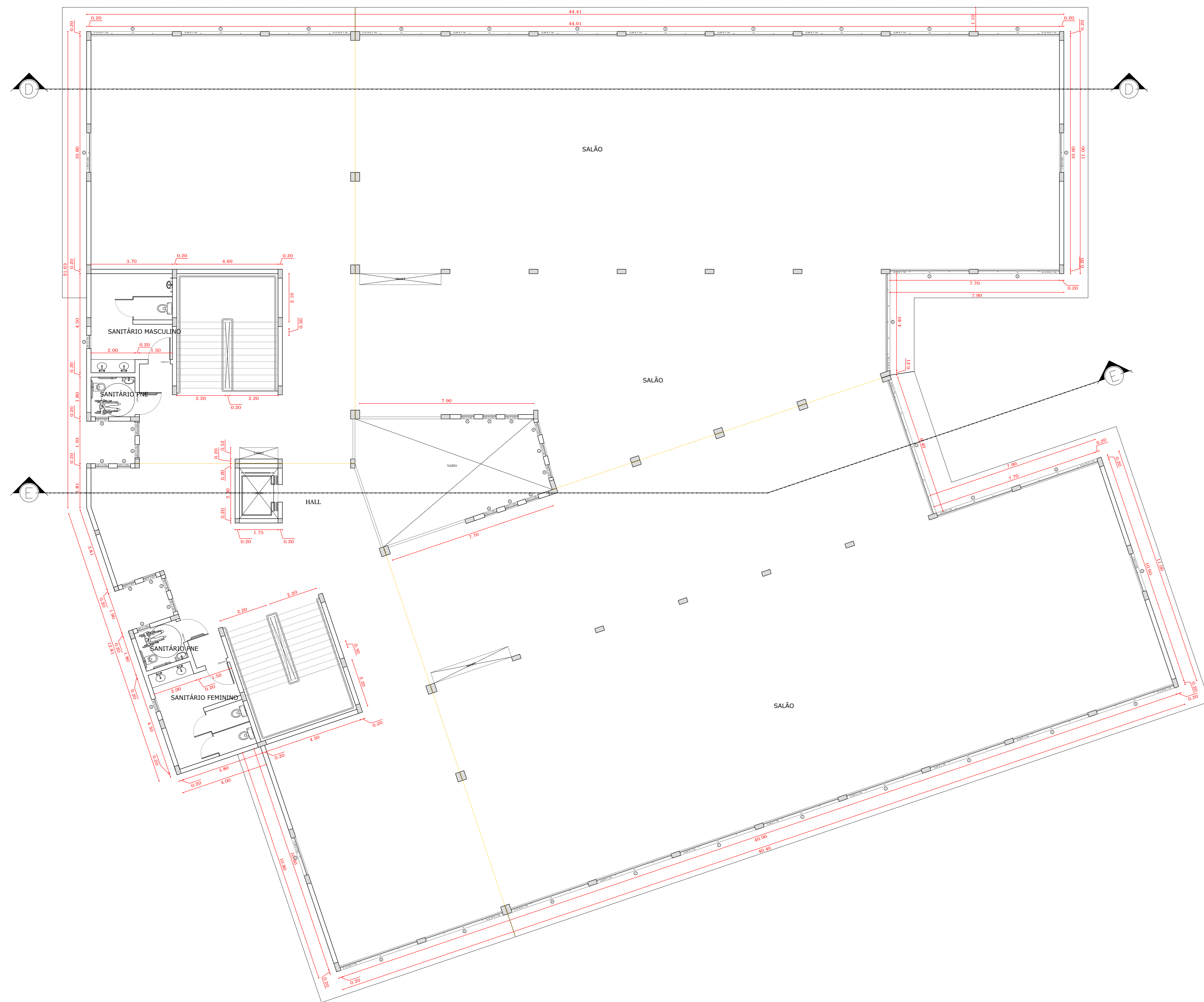
14 PISO 5 ESCALA 1:100
