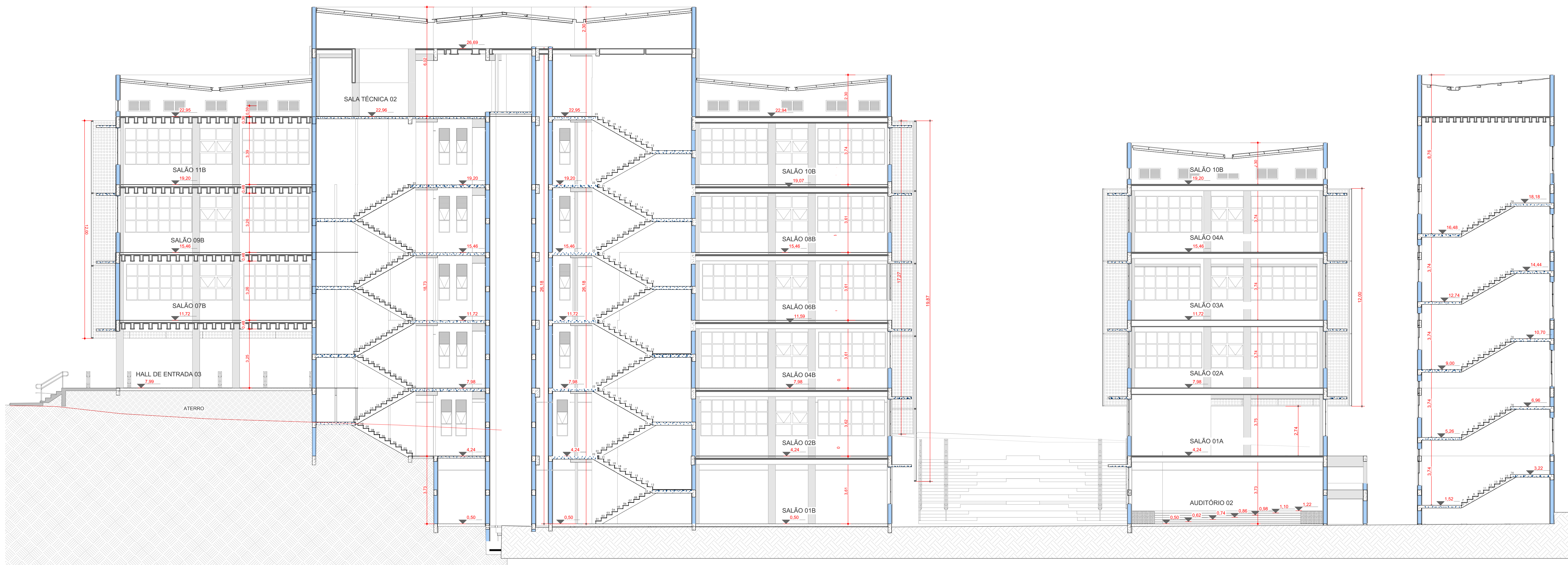
1 CORTE EE ESC. 1:100
