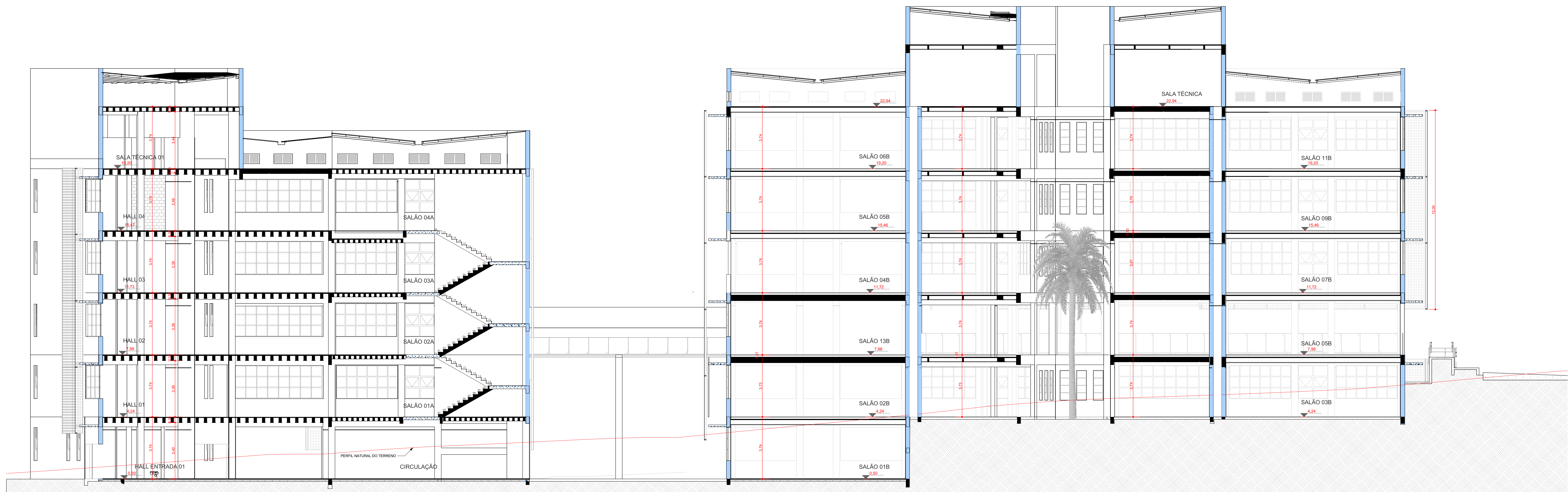
3 CORTE FF ESC. 1:100
