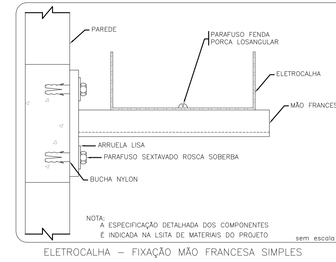
ELETROCALHA - FIXAÇÃO MÃO FRANCESA SIMPLES
