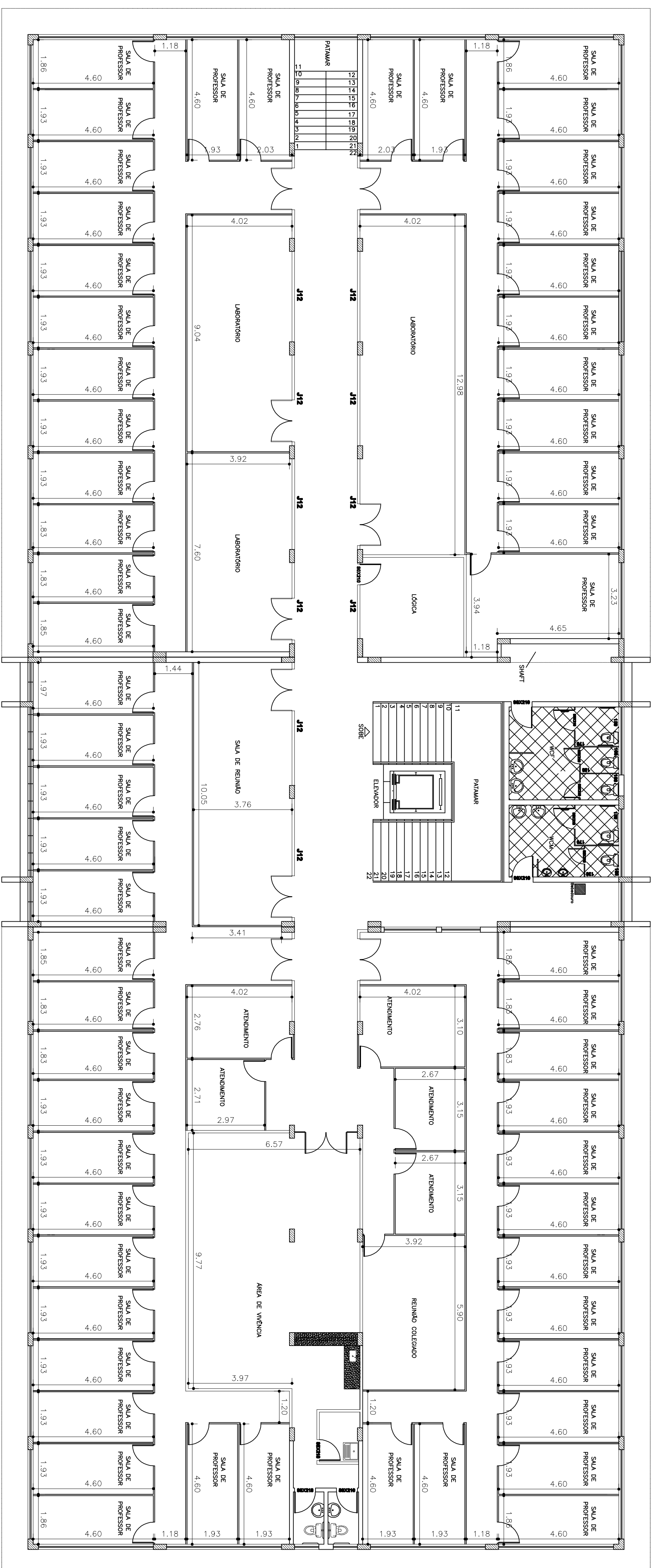
PLANTA DETALHAMENTO DIVISÓRIAS 3º PAVIMENTO ESCALA:1:100
