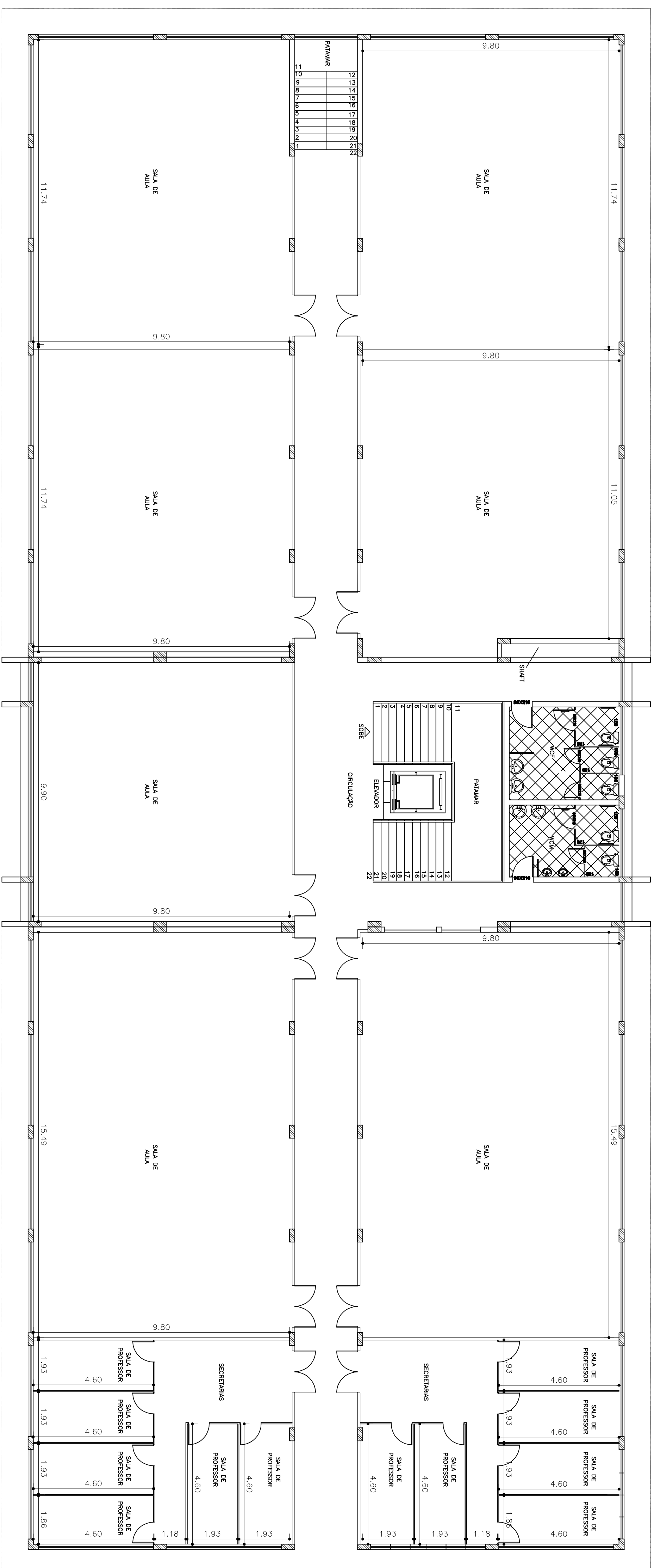
PLANTA DETALHAMENTO DIVISÓRIAS 2º PAVIMENTO ESCALA:1:100
