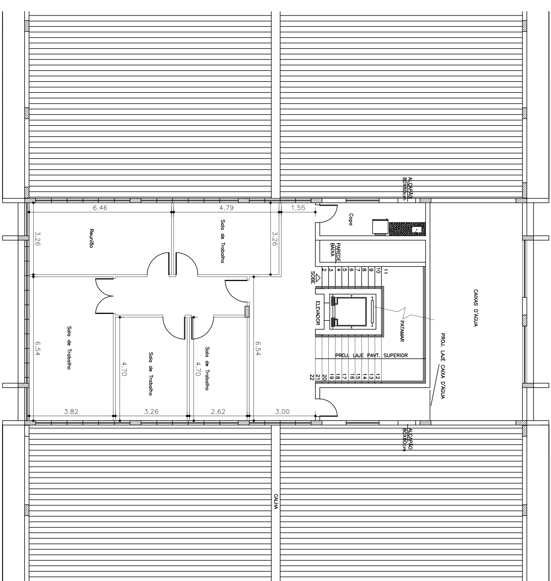
PLANTA DETALHAMENTO DIVISÓRIAS 4º PAVIMENTO ESCALA:1:100
