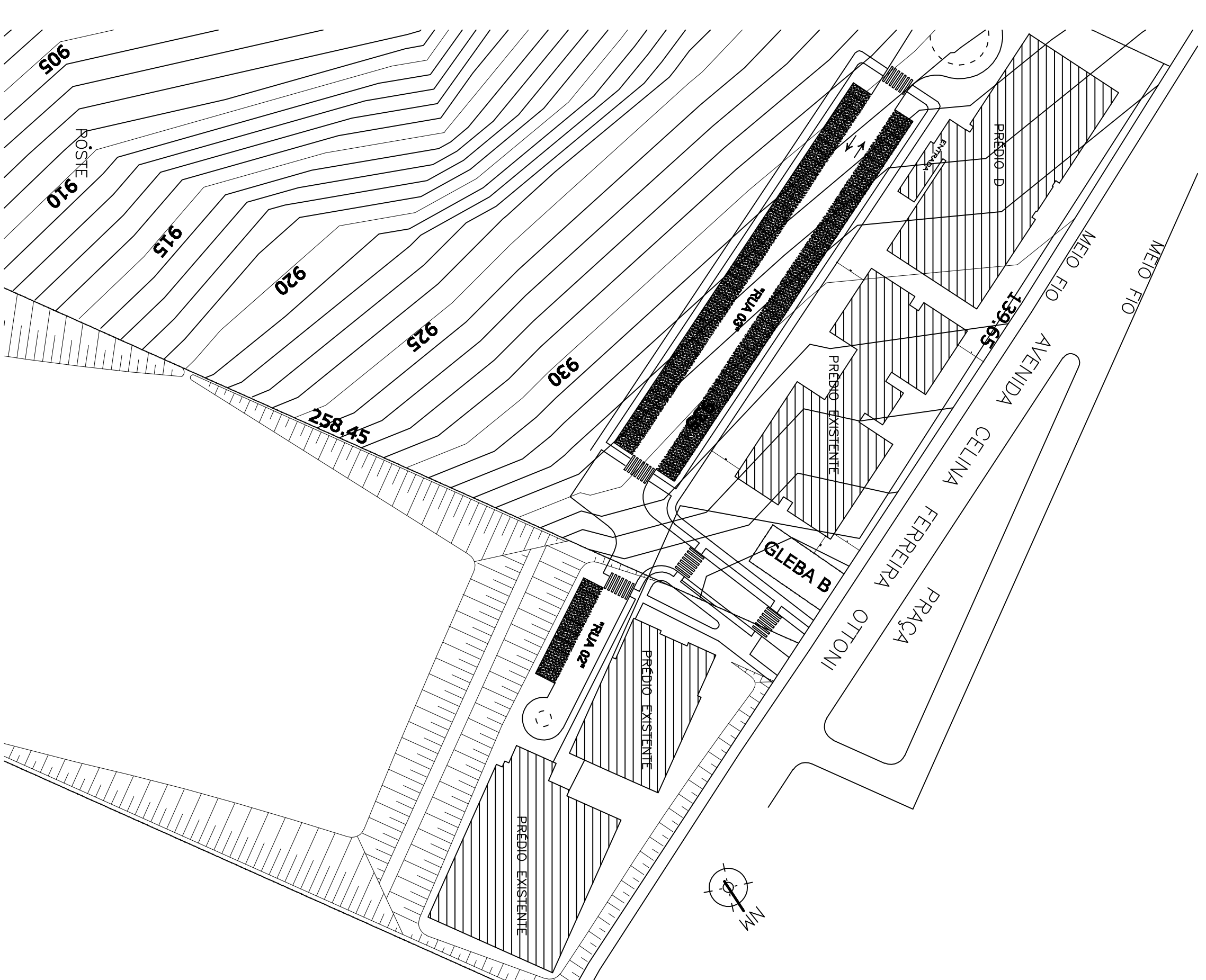
PLANTA DE SITUAÇÃO SEM ESCALA
