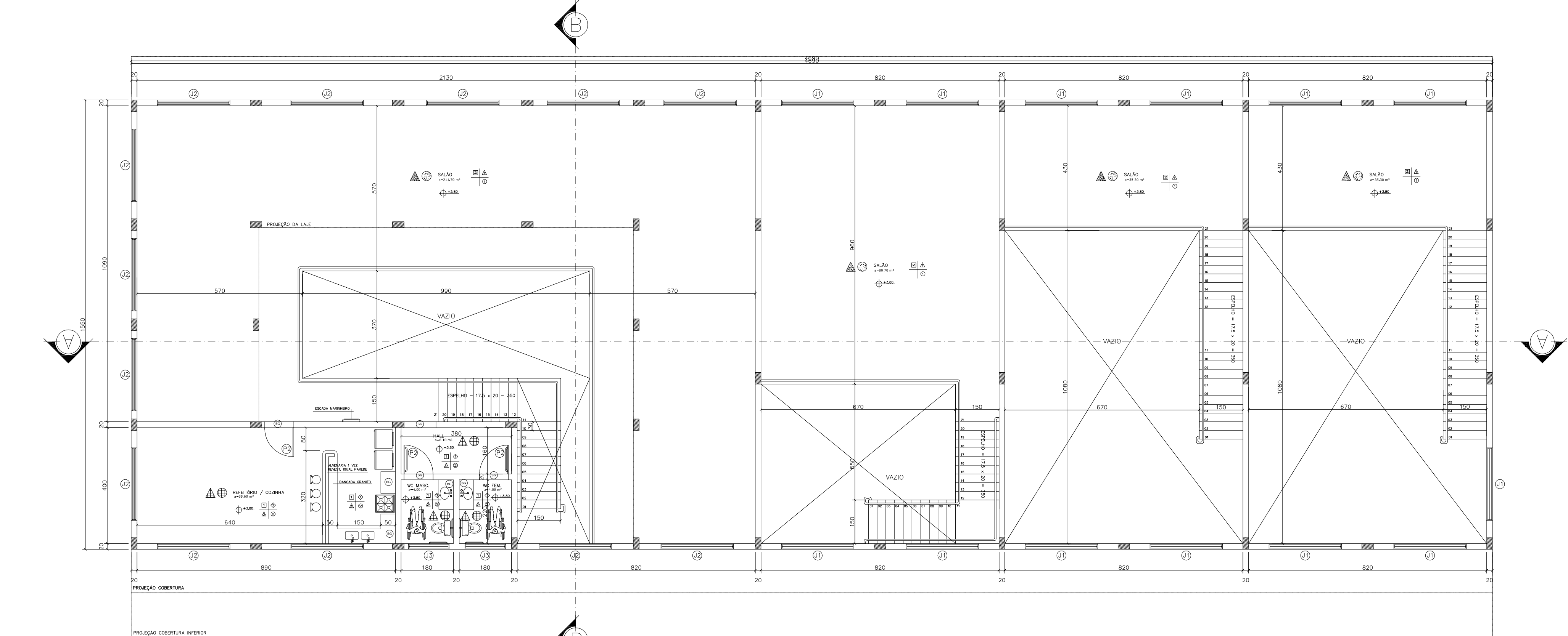
PLANTA BAIXA 1º PAVIMENTO ESC.: 1/100
