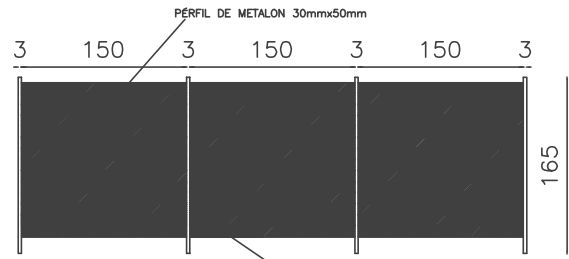
PALETAS EM CHAPA DE FERRO n°20 VISTA FRONTAL
