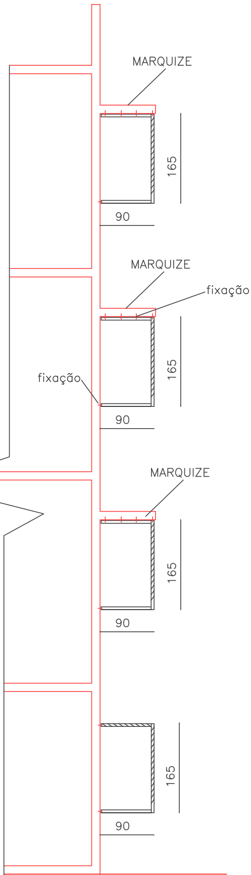
CORTE
