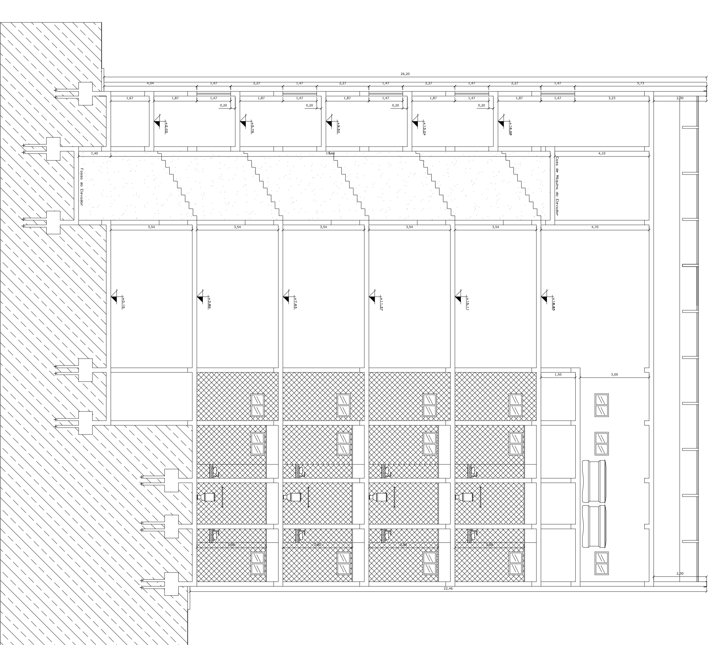
CORTE CC ESC.: 1:100
