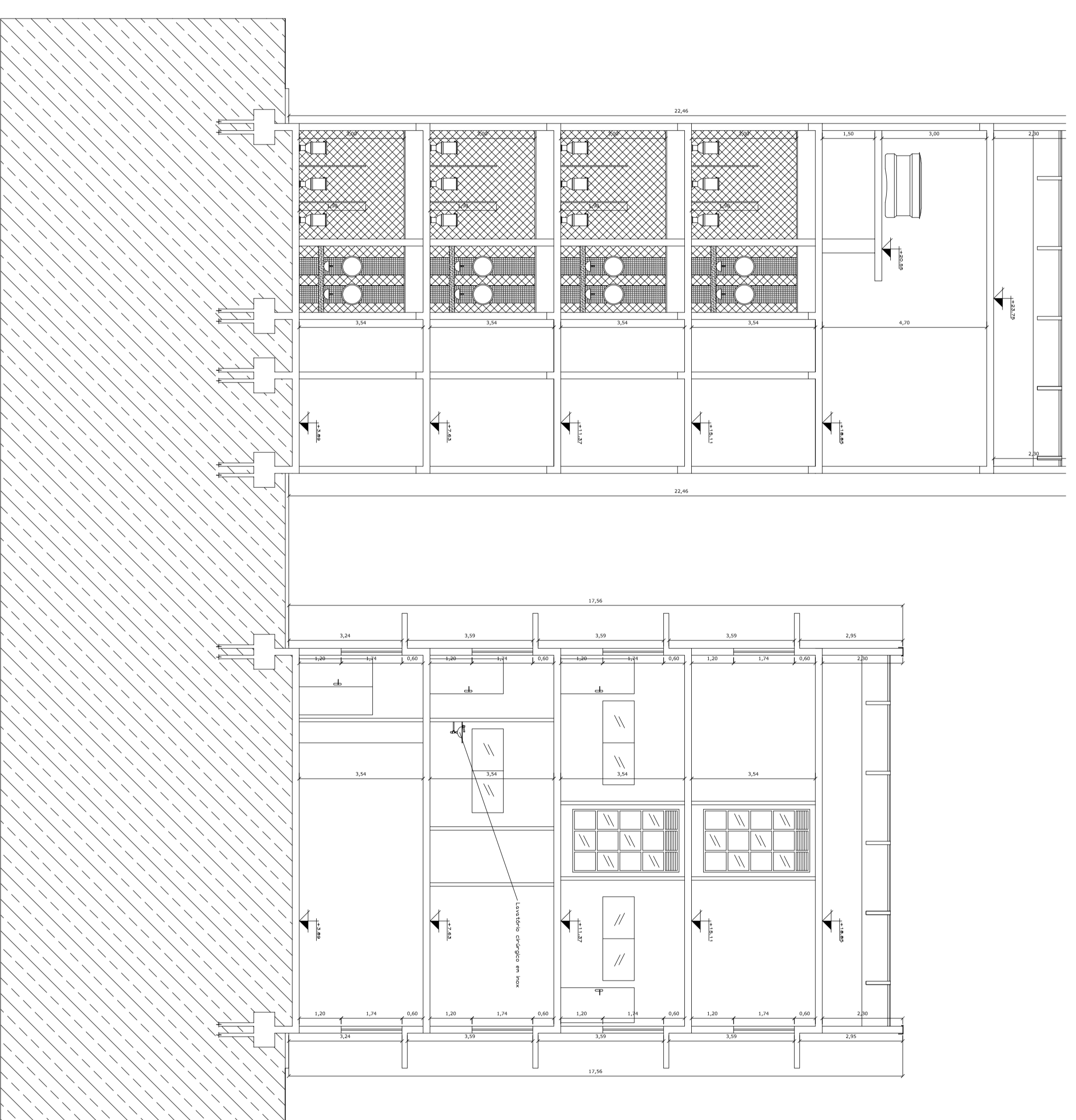
CORTE BB ESC.: 1:100
