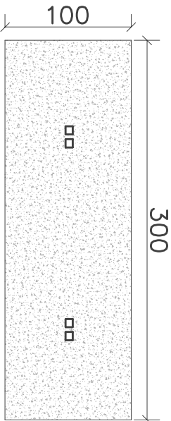
VISTA SUPERIOR
