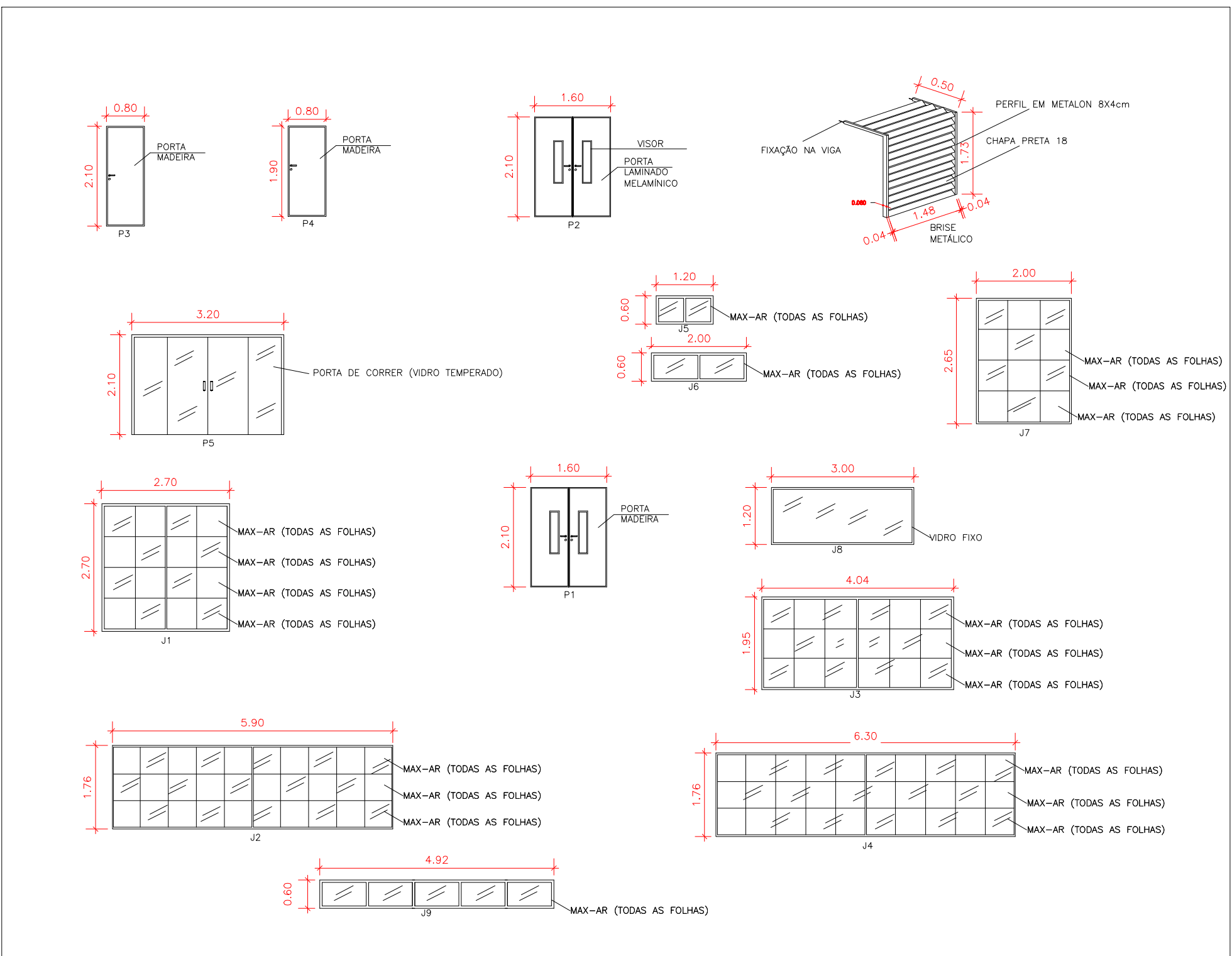
DETALHAMENTO DAS ESQUADRIAS ESCALA 1/100
