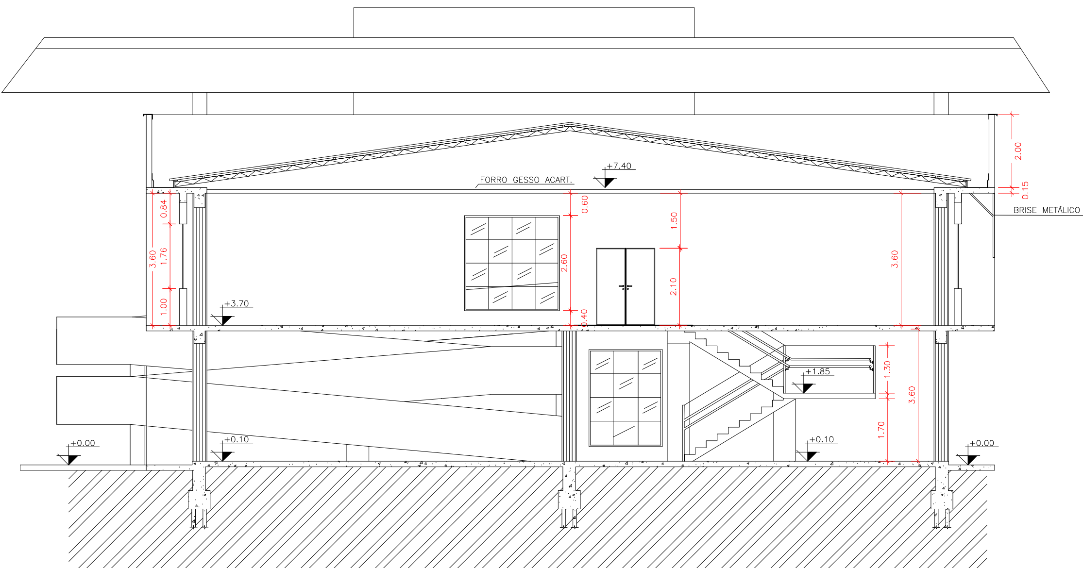
CORTE CC ESCALA 1/100
