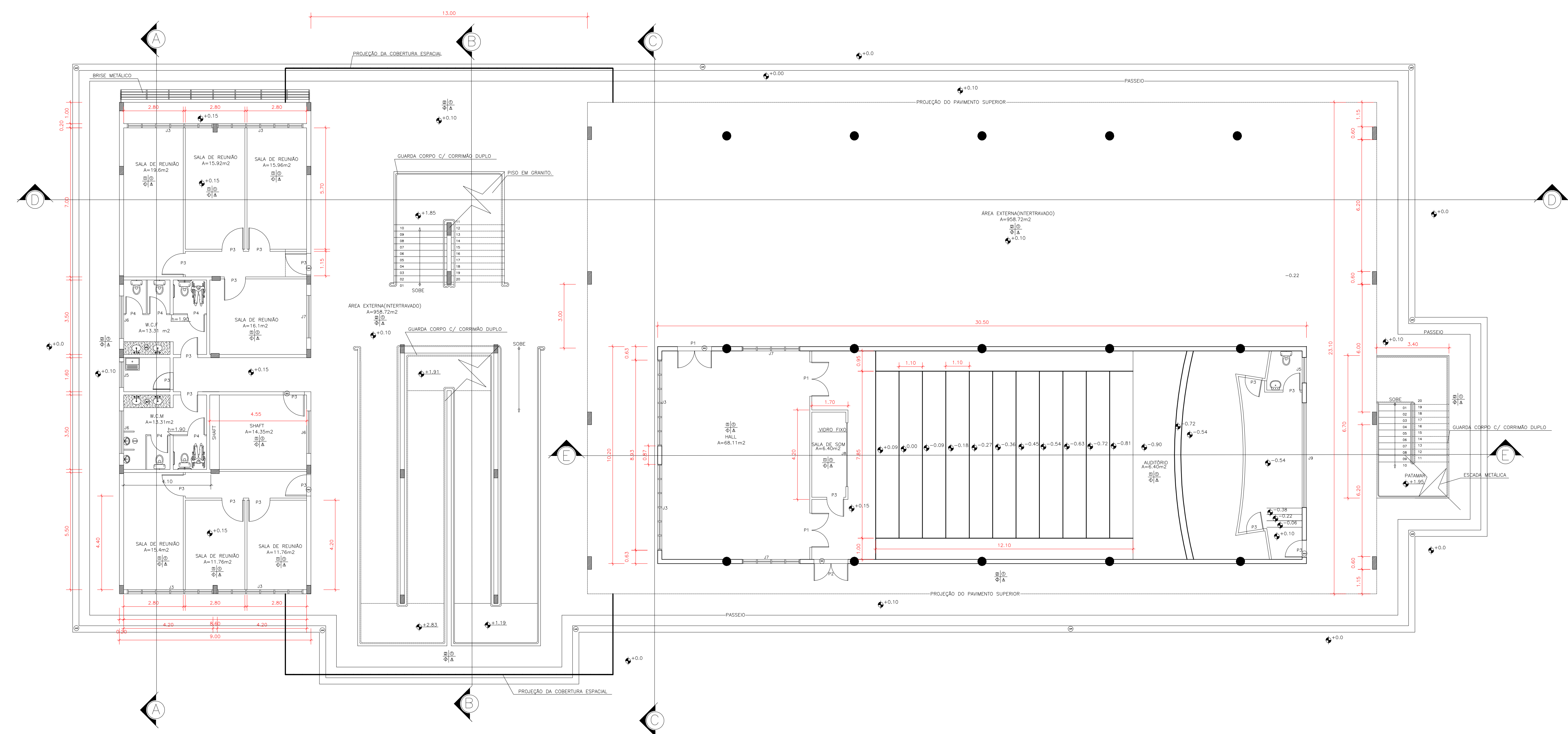
PLANTA 1º PAVIMENTO (PILOTIS) ESC.: 1/100
