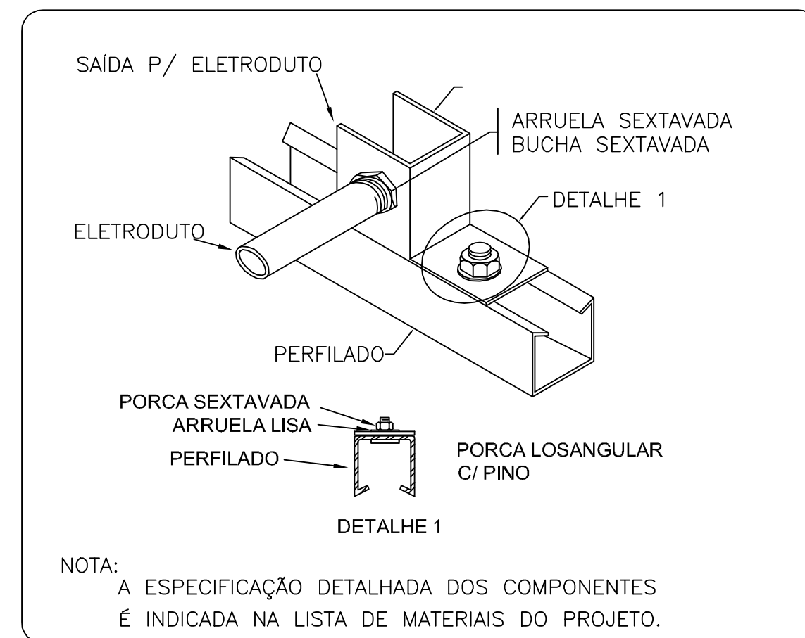
ENTRADA E SAÍDA DE ELETRODUTO EM PERFILADO
