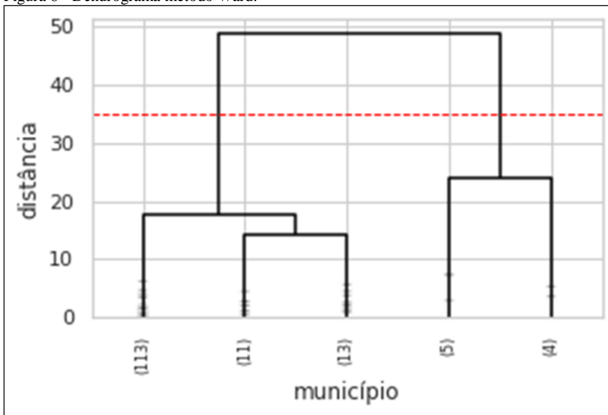
Figura 6 - Dendrograma método Ward.
