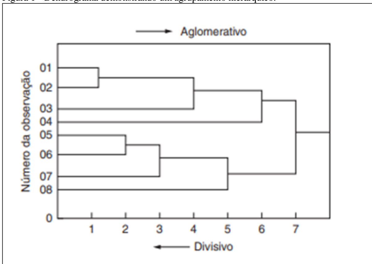
Figura 1 - Dendrograma demonstrando um agrupamento hierárquico.
