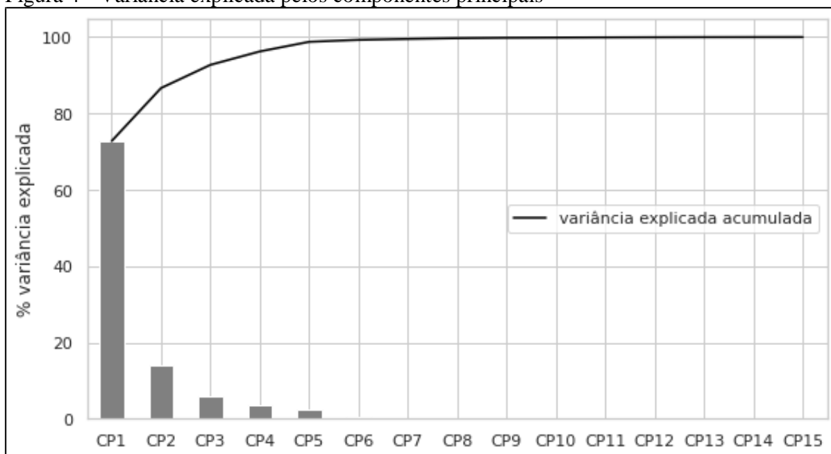
Figura 4 - Variância explicada pelos componentes principais
